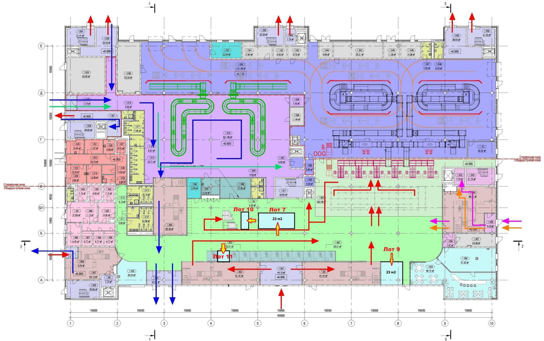
План функционального зонирования 1-го этажа (на отм. 0.000)
